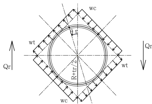
図 3-3-1. 梁断面
