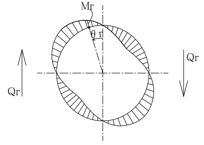
図 3-3-4. Q_r により生ずる OS リング肉内の曲げモーメント分布
