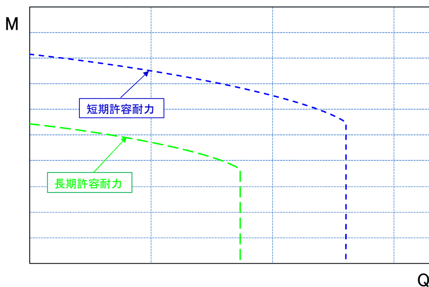
図 3-2-12.本工法_MQ 耐力曲線
