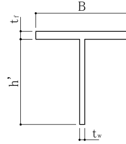
図 3-3-7. T 形断面部分
