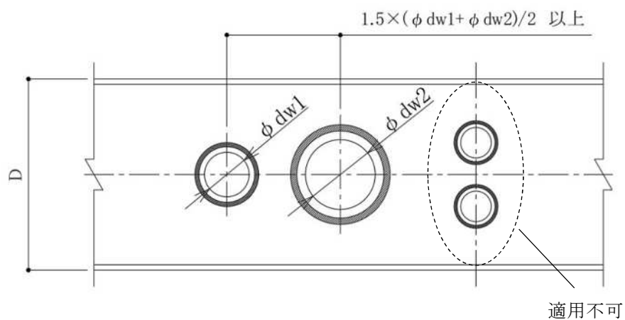
図 3-2-3.本工法の適用範囲-3
