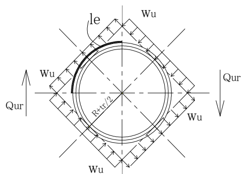
図 3-3-10. すみ肉溶接部に作用する等分布荷重
