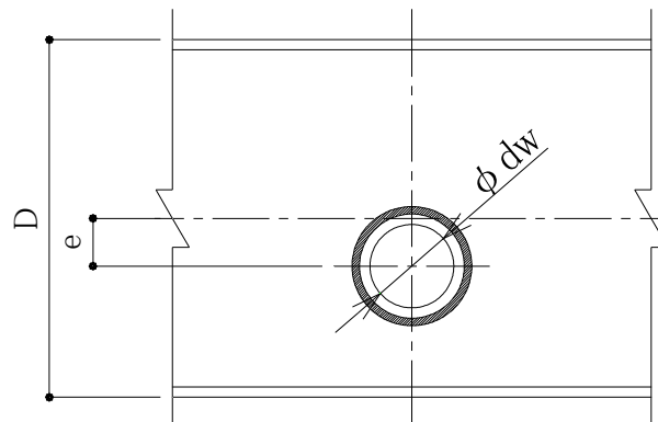
図 3-2-2.本工法の適用範囲-2
