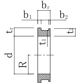
図 3-3-5. OS リング断面
