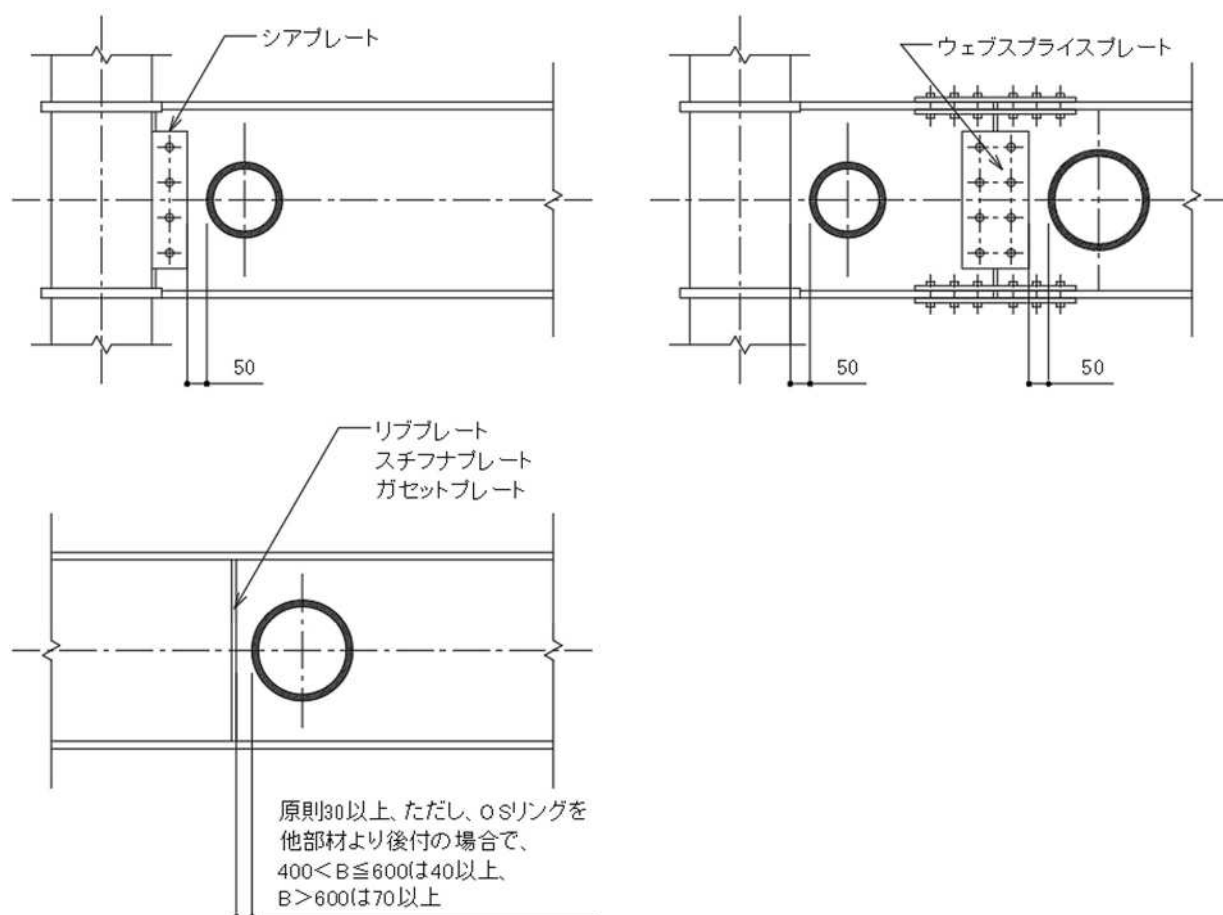
図 3-2-5. 本工法の適用範囲-5
