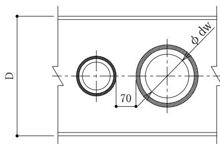
図 3-2-6. 本工法の適用範囲-6
