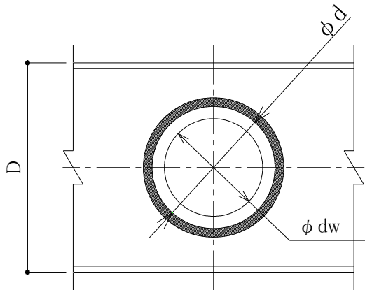
図 3-2-1.本工法の適用範囲-1
