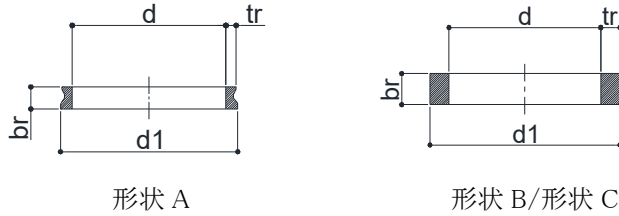
図 2-2-1.OS リングの形状寸法
