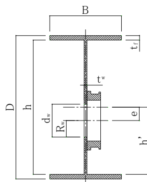
図 3-3-1. 梁断面
