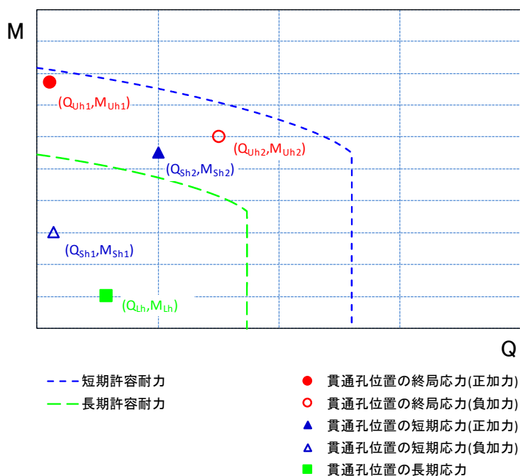
図 3-2-14.MQ 耐力曲線と存在応力 (はりの部材種別が FC or FD、鋼種が SN400A の場合)
