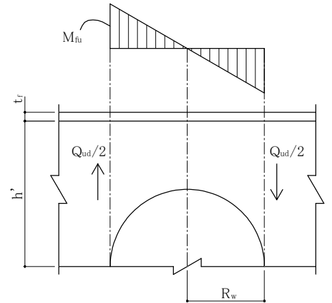
図 3-3-6.せん断力による 2 次曲げ
