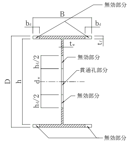
図 3-3-8 梁断面
