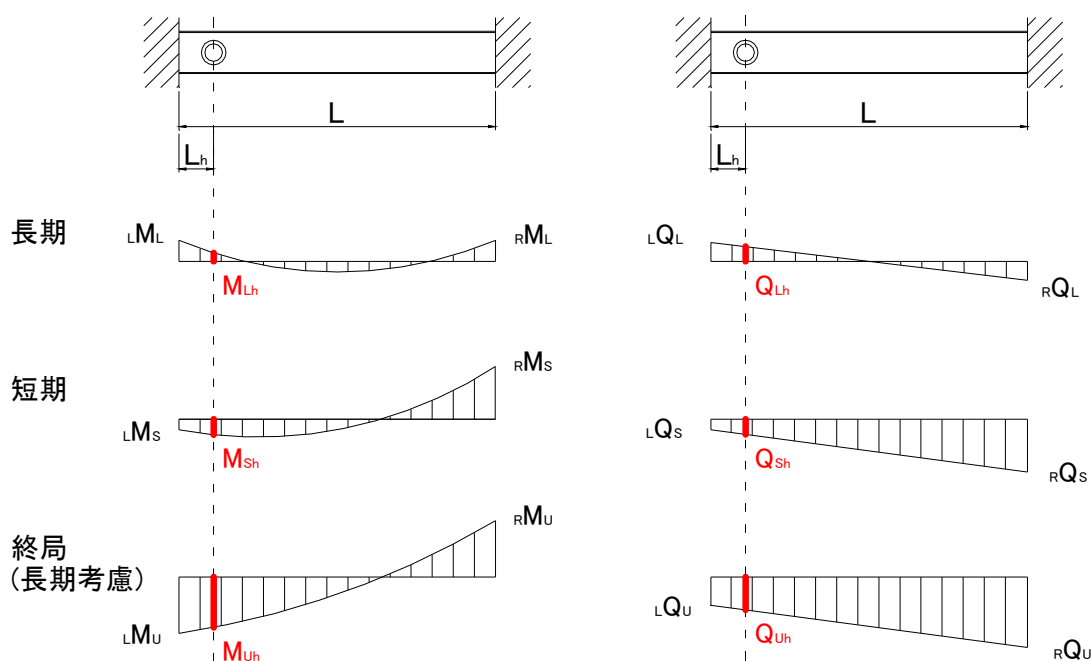
図 3-2-10.貫通孔位置の存在応力(曲げモーメント・せん断力)概要図
