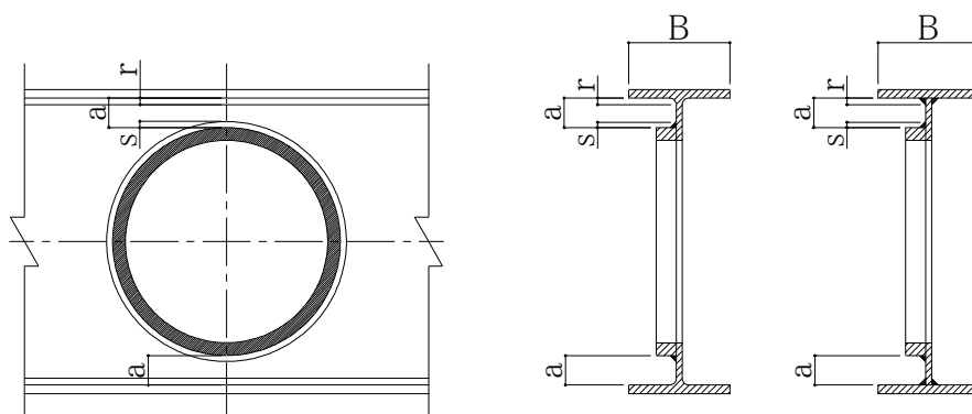
図 3-2-7. 本工法の適用範囲-7
