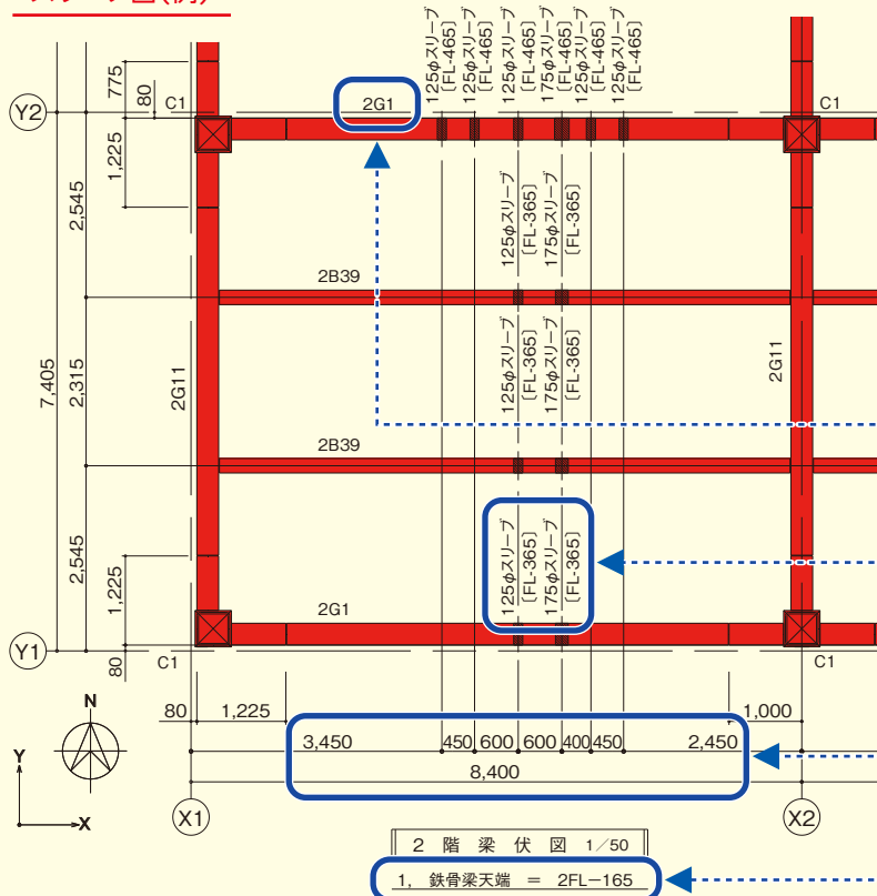
スリーブ図(例)
