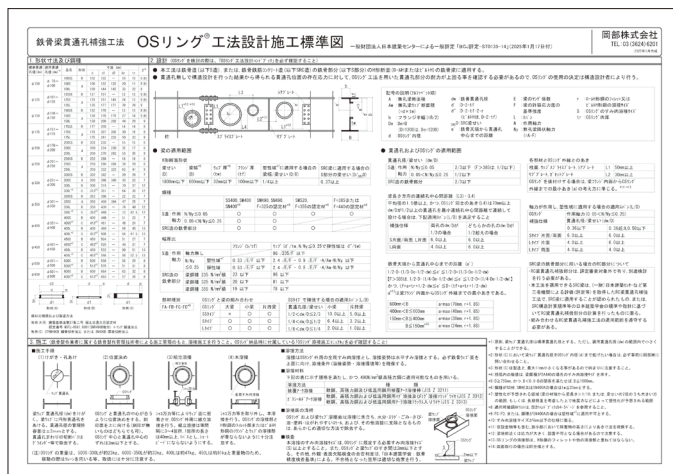
OSリング設計施工標準
