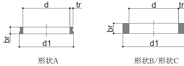
図2-2-1 OSリングの形状寸法
